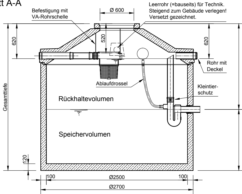
Schnitt A-A
